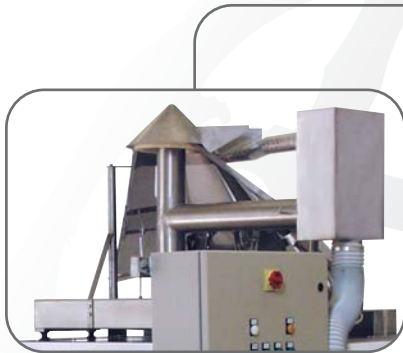
Versione speciale con cono spanditore per trafila circolare
